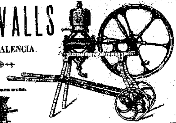
Bomba sistema Lapoyre Cilindro, eje y ruedas de metal. N.º 1. Renda. por hora 5,000 l. Ptas. 350. N.º 2. " " 8,000 l. " 450.
