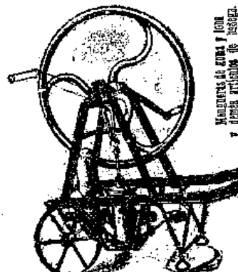
Bomba LA EXCELENTE. Cilindro, eje y ruedas de metal. N.º 1. 6,000 l. 1 volante. Ptas. 325. N.º 2. 8,000 l. 1 id. " 375.
